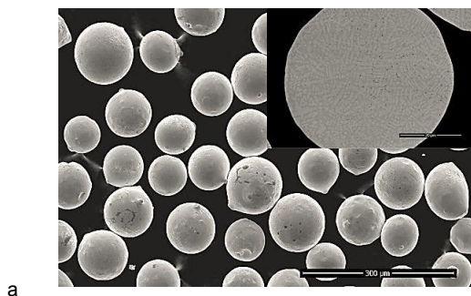
Fig. 1 - Morphology of Metco 12C powder and EDX spectrum of a single powder particle Morfologia pudrei Metco 12C și spectrul EDX obținut în cazul unei singure particule.
