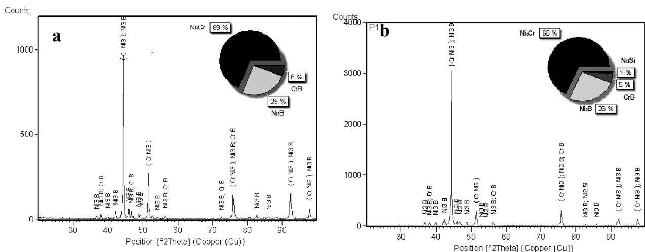
Fig. 3 - XRD of feedstock powder (a) and cladded coating (b) / Difractogramele obținute în cazul pudrei utilizate (a) și a straturilor obținute (b).
