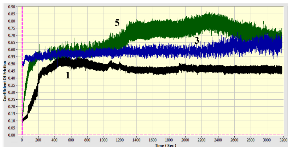
Fig. 4 - CoF function of sliding time of NiCrBSi laser cladded coatings for samples 1, 3 and 5 / CoF funcție de timpul de alunecare pentru straturile NiCrBSi ale probelor 1, 3 și 5.
