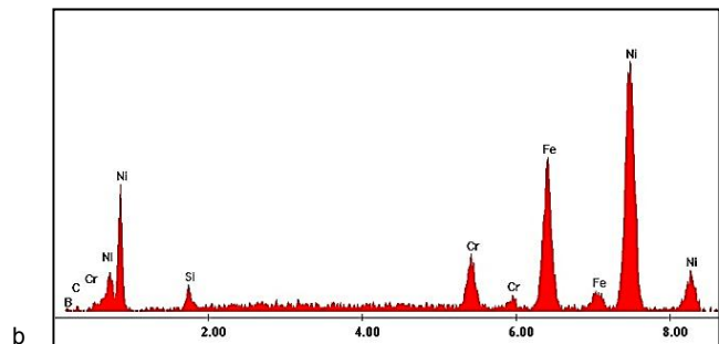
Fig. 1 - Morphology of Metco 12C powder and EDX spectrum of a single powder particle Morfologia pudrei Metco 12C și spectrul EDX obținut în cazul unei singure particule.
